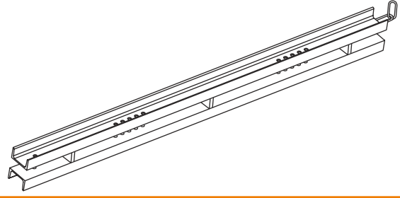
Kuşak Birleştirme Elemanı / Waler Coupler
