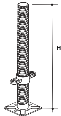
Ayarlanabilir Alt Ayar Mili / Adjustable Base Plate
